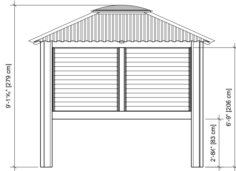
Élévation avant
