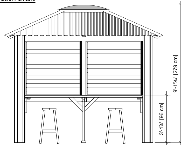
Élévation avant
